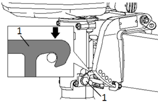
1.Tilt lock
